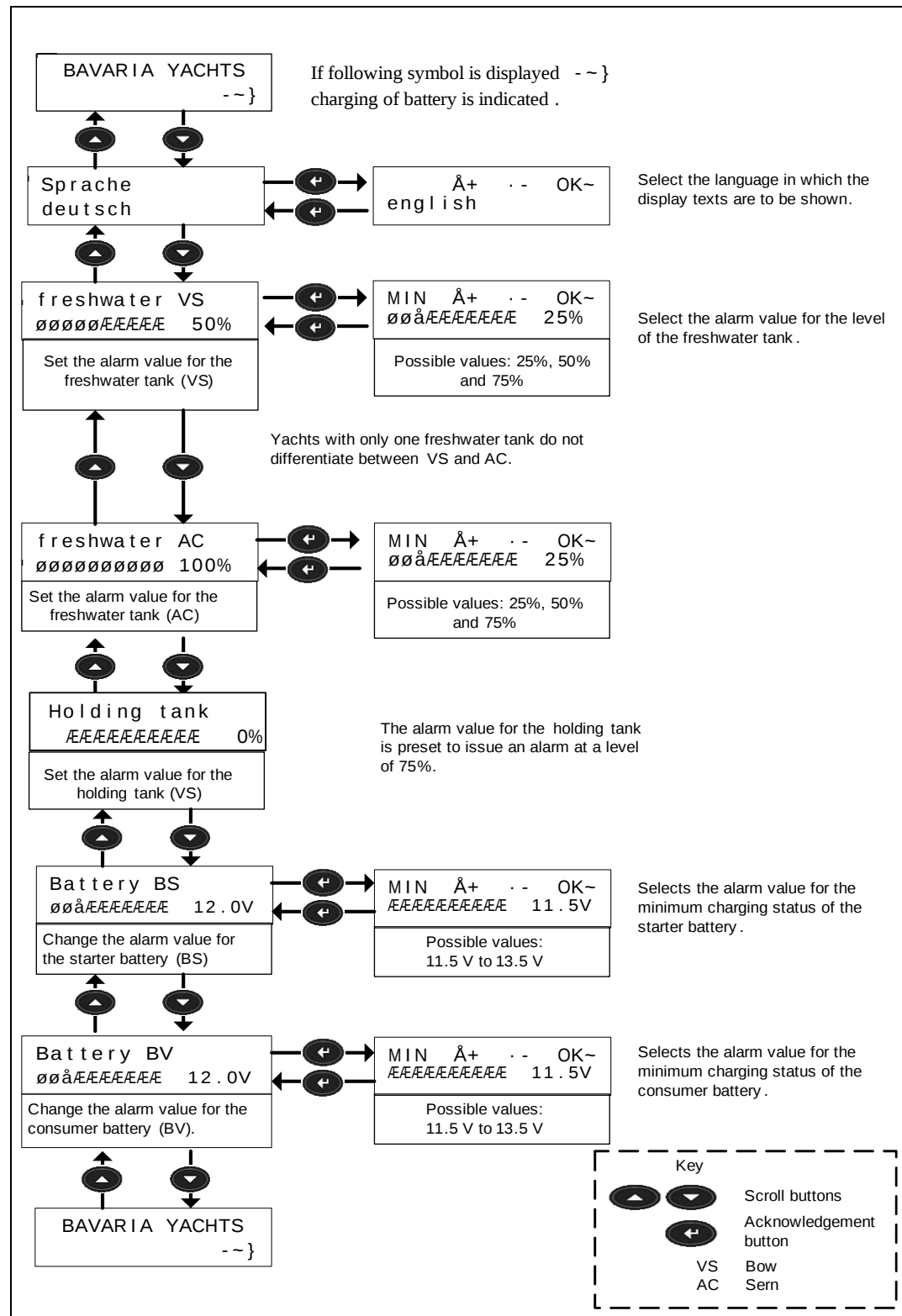
Fig. 4 Panel 301 menu
