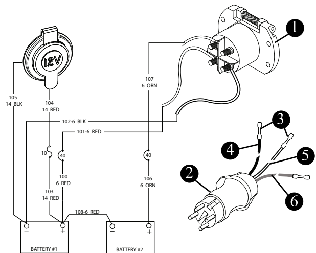
12V/24V WIRING DIAGRAM
