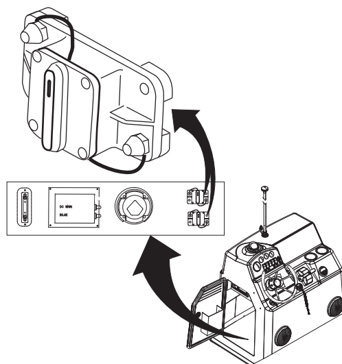
Trolling Motor Receptacle Breakers Fig. 4.4.1
