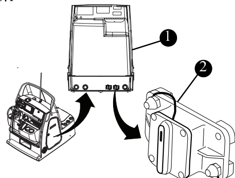
Trolling Motor Receptacle Breakers Fig. 4.3.1
