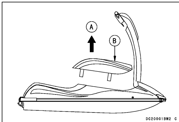
A. Pull up
