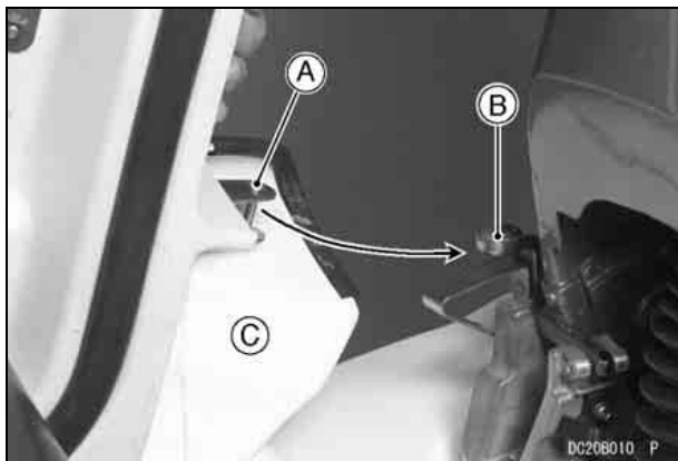
A. Hood Hook B. Bracket
