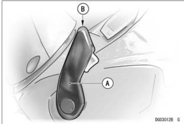
A. Shift Lever B. "R" position
