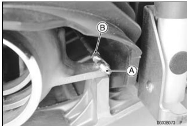
A. Joint B. Locknut
