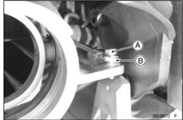
A. Bolt B. Joint
