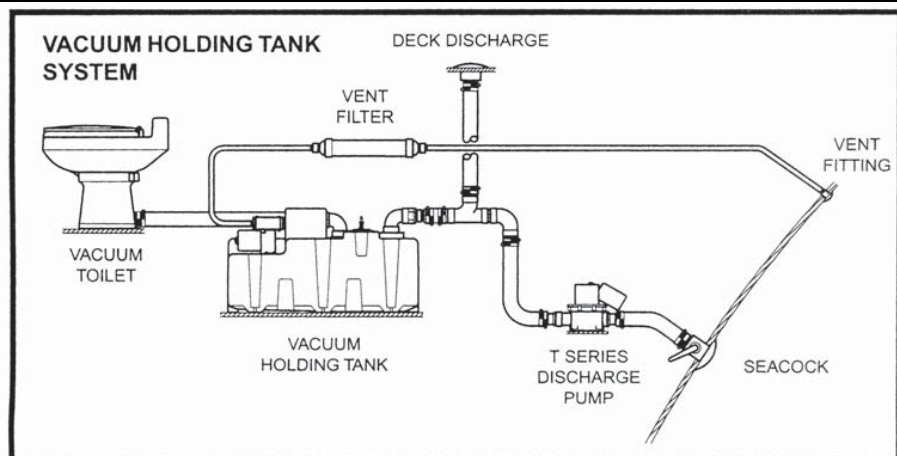
VacuFlush Head
