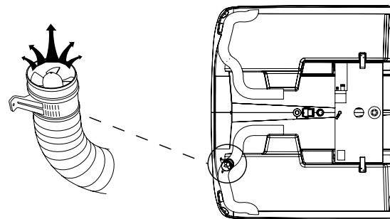
BILGE BLOWER (FIG. 16.3)
