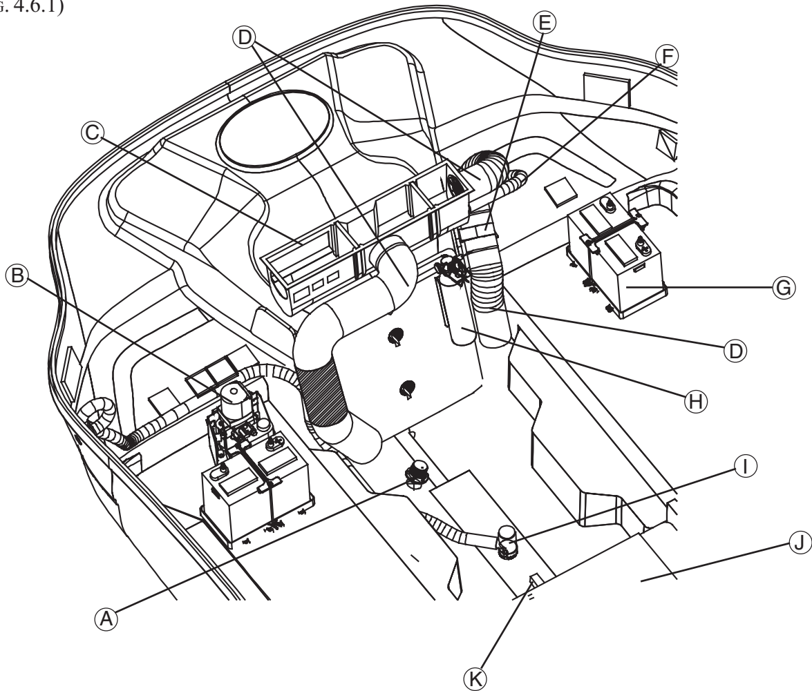
BILGE LAYOUT (FIG. 4.6.1)
