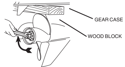
PROPELLER (FIG. 4.5.2)
