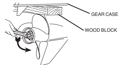
PROPELLER (FIG. 4.4.2)
