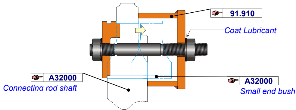
Fig.6 Removal device for small end bush (소단부 부시용 분해 공구)
