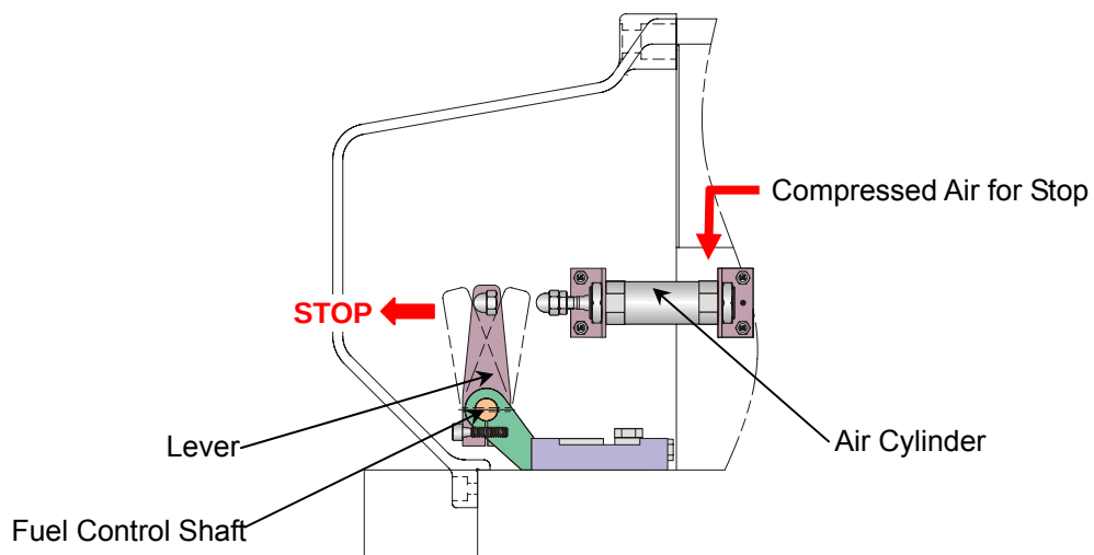
Fig. 5 Mechanical fuel limiter for starting (시동용 기계적 연료 제한 장치)
