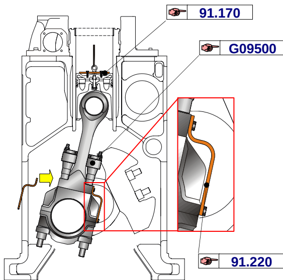
Fig.1 Loosening of the nuts for connecting rod studs (커넥팅 로드 스터드용 너트 분해)
