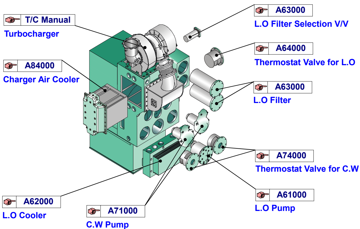
Fig. 2 Equipments for feed module (피드 모듈 장치)
