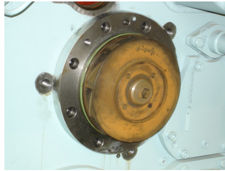
Fig.12 Assembly of C.W.Pump housing( 청수 펌프 하우징 조립)
