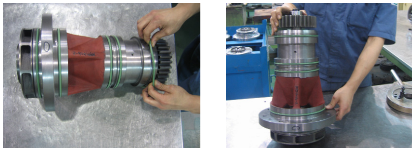
Fig.11 Insertion of O-ring and end products (오링 조립과 완제품)
