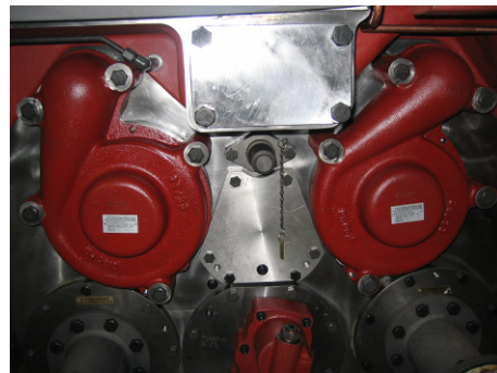
Fig.13 Assembly of C.W.Pump cover and the assembled C.W.Pump (청수 펌프 커버 조립과 청수 펌프 조립완료된 상태)
