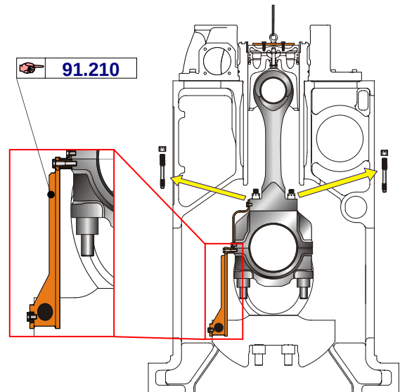
Fig.2 Installing of turning bracket (회전 방지구의 설치)
