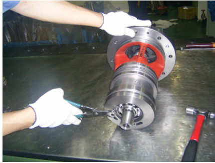
Fig.6 Assembly of snap ring into pump housing (펌프 하우징에 스냅 링 조립)
