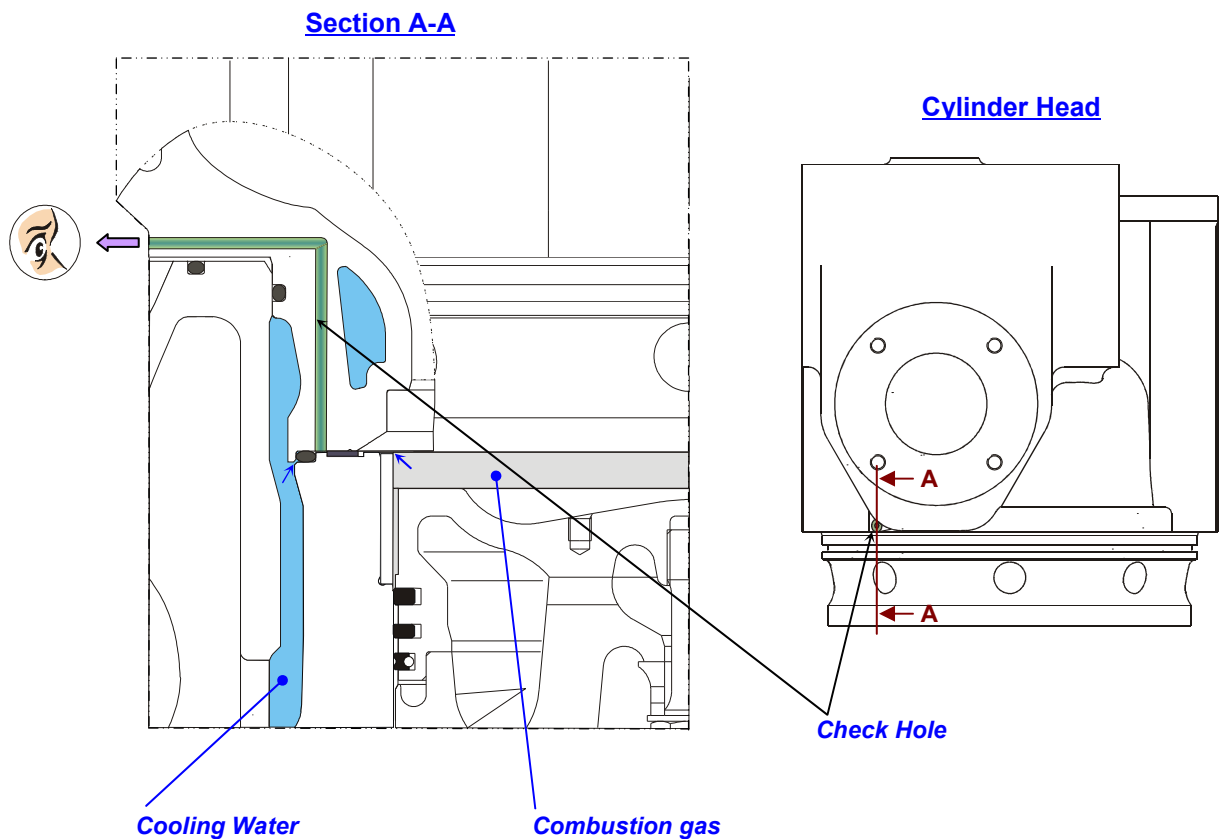
Fig.2 Check hole in cylinder head (실린더 헤드 점검 홀)
