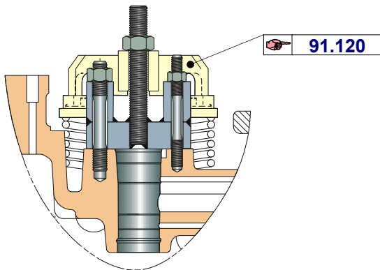
Fig. 1 Mounting of tool (공구의 설치)
