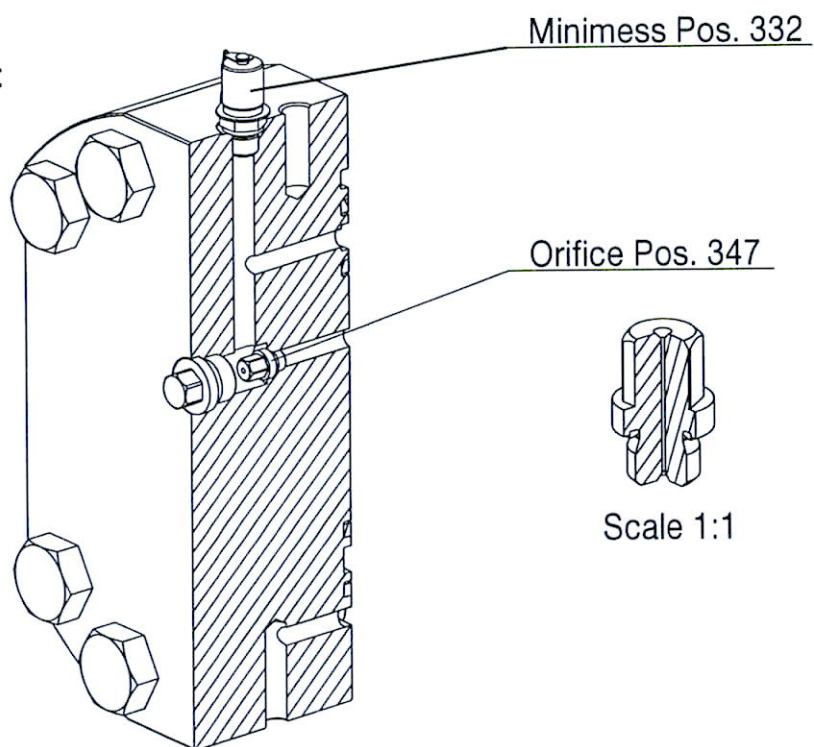
Fig. 2 End Flange:
