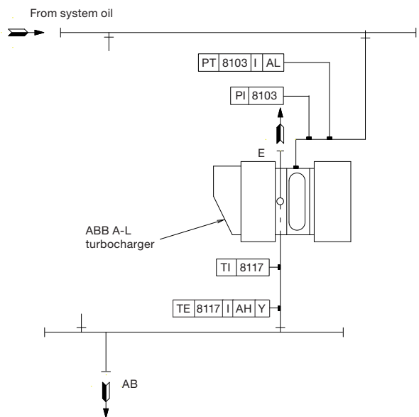
Fig. 8.03.03: ABB turbocharger type A-L
