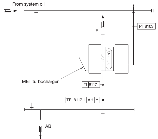
Fig. 8.03.02: Mitsubishi turbocharger type MET
